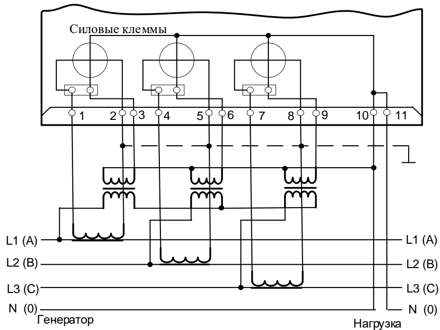
Рисунок 4 - Схема подключения счетчика в корпусе 10м к трехфазной четырехпроводной сети с использованием трансформаторов тока и напряжения
