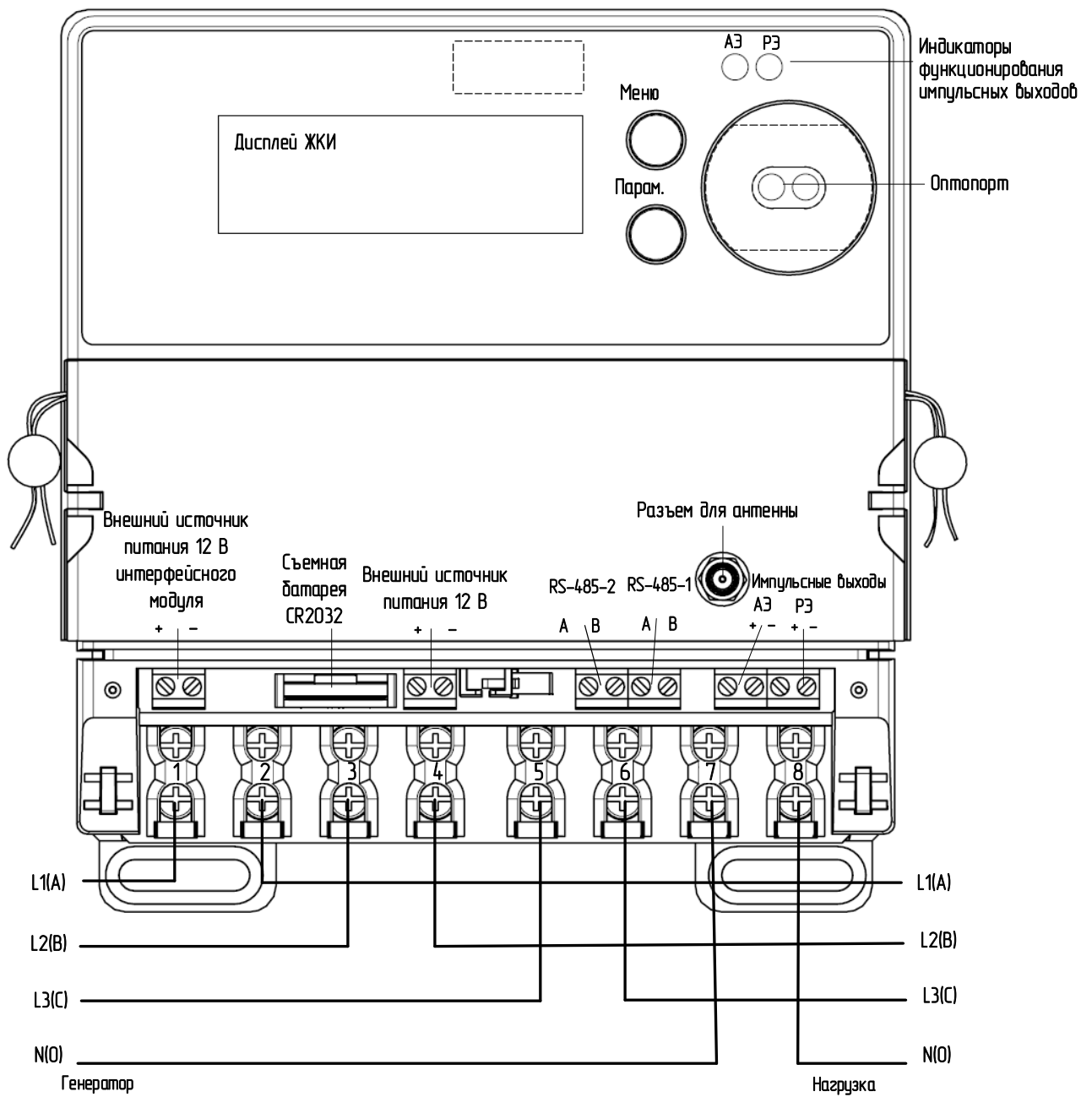
Рисунок 3 - Внешний вид, органы управления и назначения клемм счетчика в корпусе 10м с расширенным функционалом непосредственного включения
