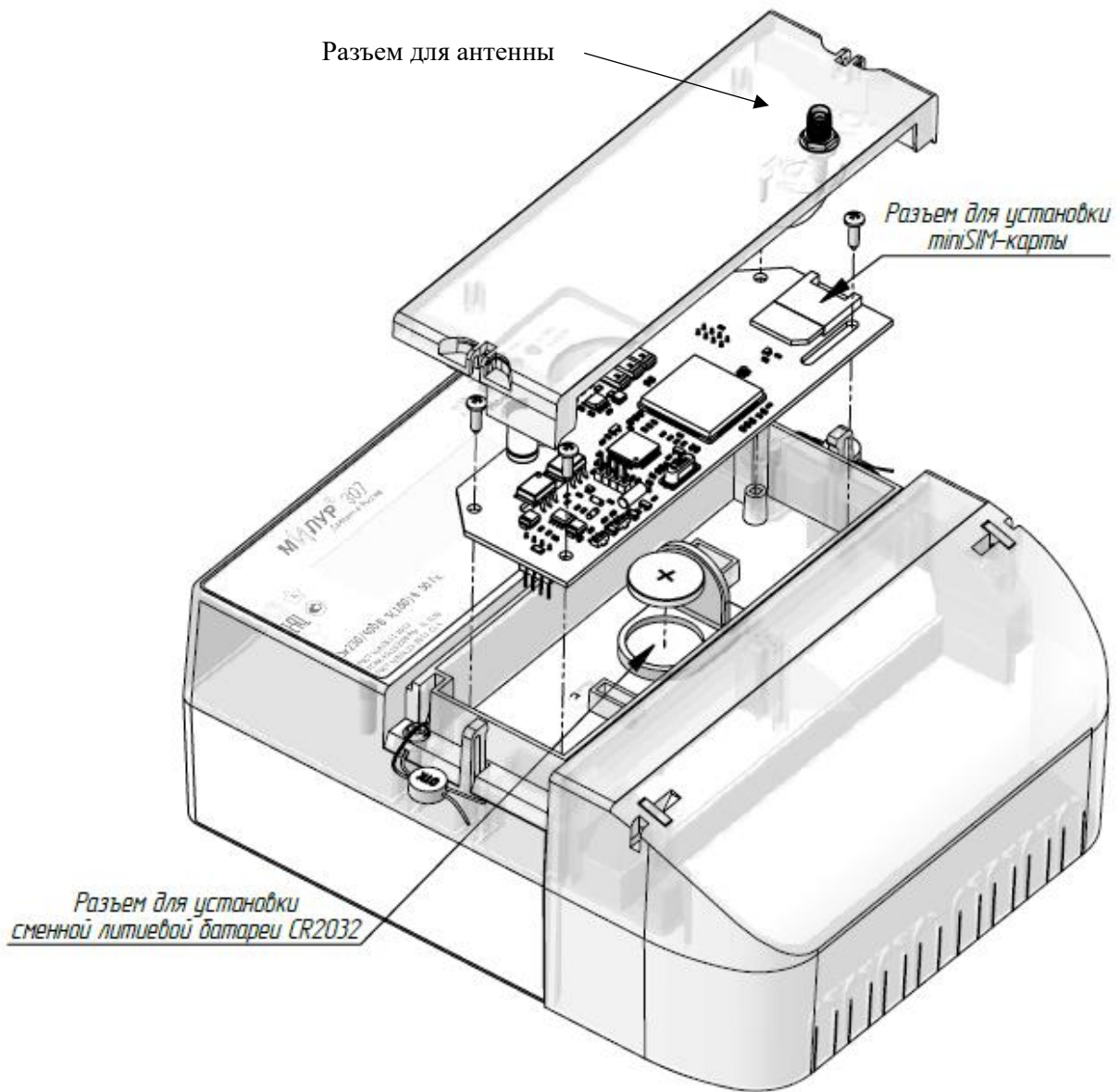
Рисунок 18 - Расположение батареи CR2032 и SIM-карты в счетчике в корпусе 10м трансформаторного включения
