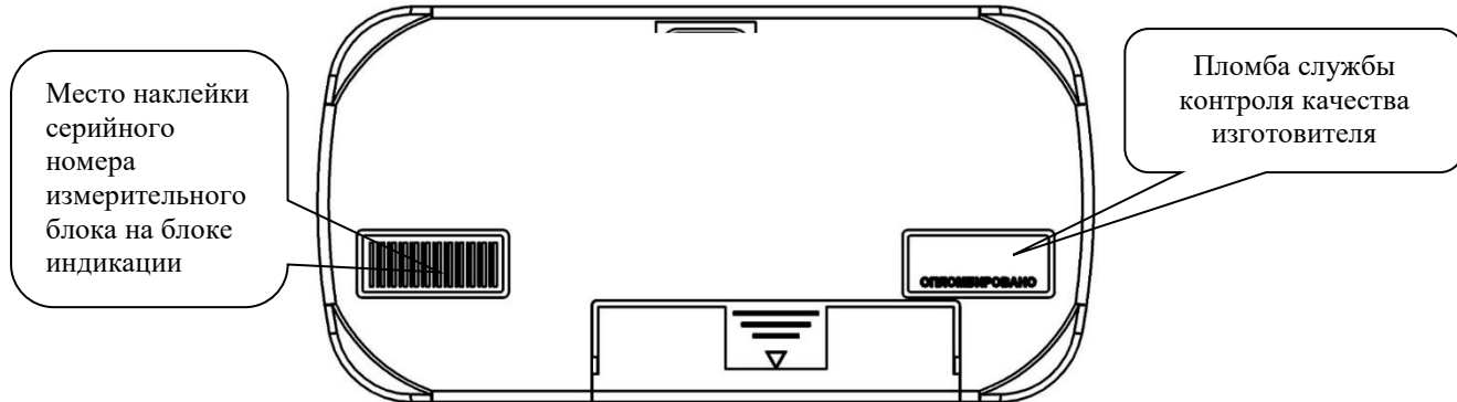
Рисунок 14 - Схема пломбировки блока индикации Милур Т и место наклейки серийного номера измерительного блока, к которому прикреплен блок индикации
