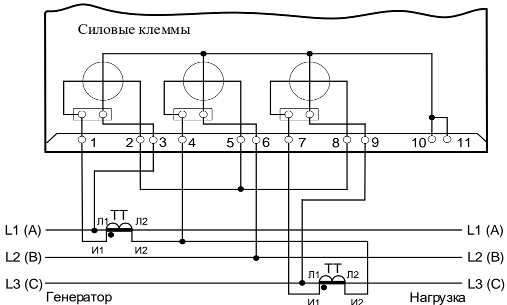
Рисунок 5 - Схема подключения счетчика в корпусах 9мТН35 и 10м к трехфазной трехпроводной сети с помощью двух трансформаторов тока
