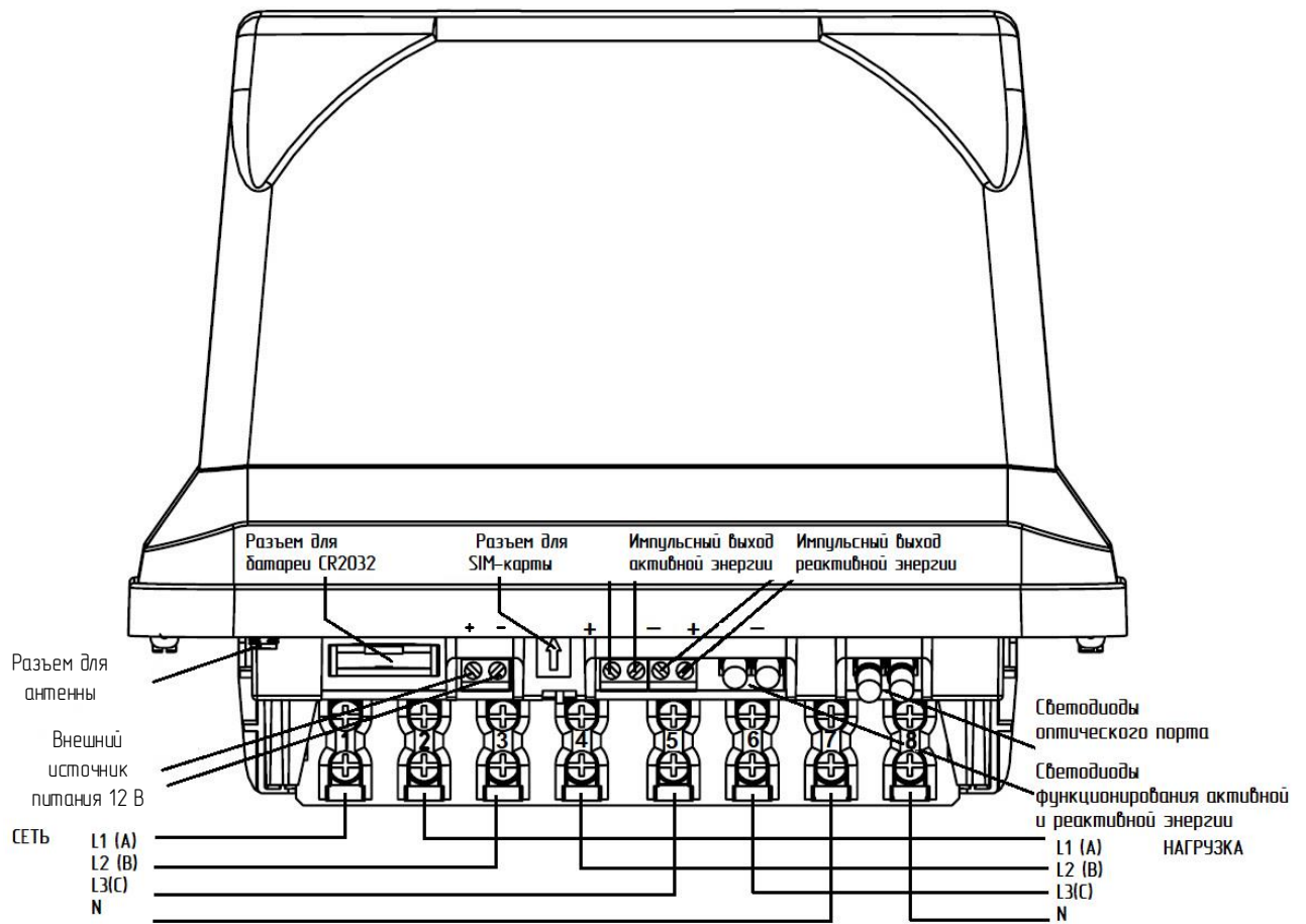
Рисунок 9 - Внешний вид и назначения клемм счетчика в корпусе SPLIT
