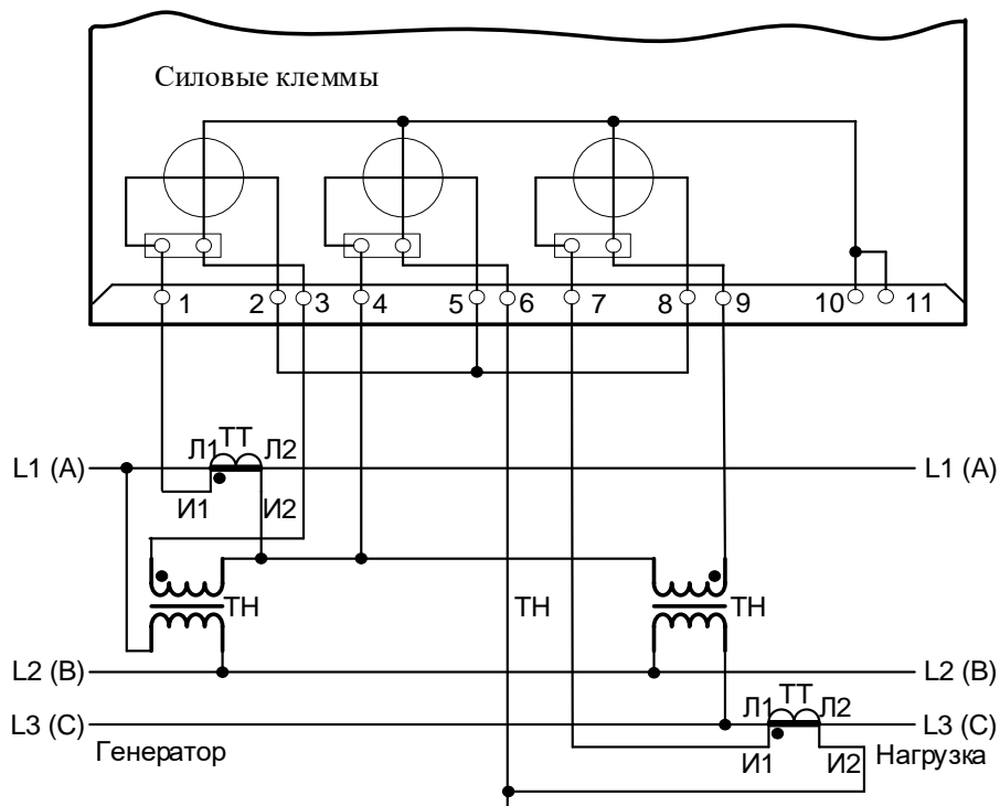
Рисунок 7 - Схема подключения счетчика в корпусе 10м к трехфазной трехпроводной сети с помощью двух трансформаторов напряжения и двух трансформаторов тока
