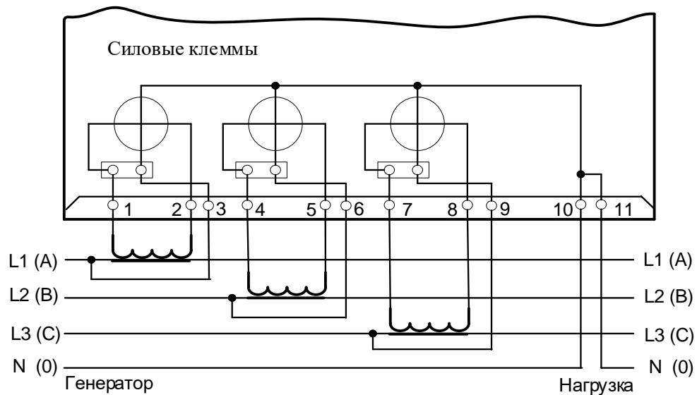
Рисунок 2 - Схема подключения счетчика в корпусе 9МТН35 к трехфазной четырехпроводной сети с использованием трансформаторов тока
