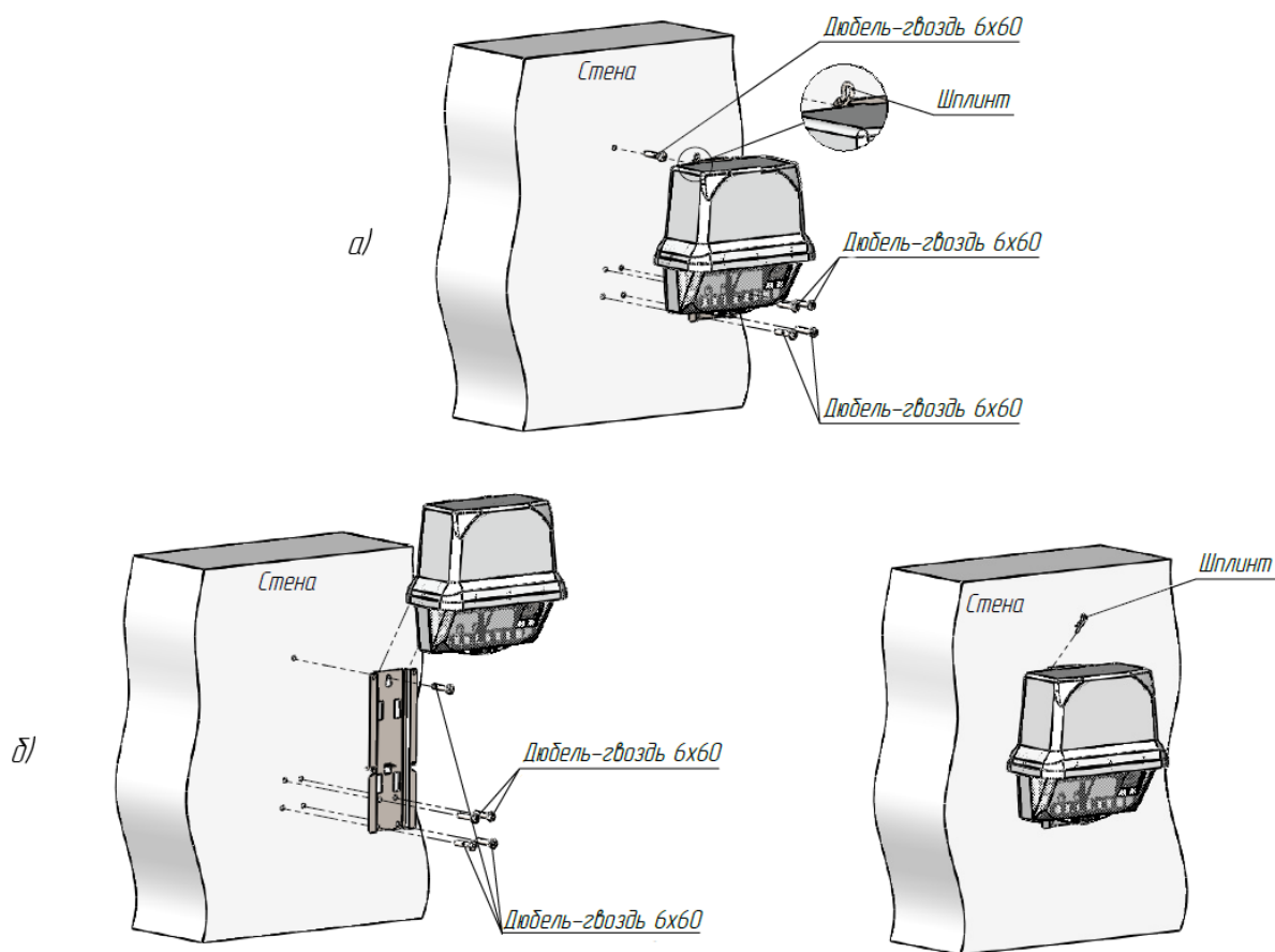
Рисунок 24 - Вариант установки счетчика в корпусе SPLIT на стену строения (два варианта)
