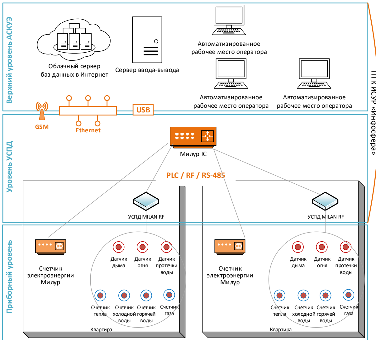
Рисунок 27 - Построение ИСУЭЭ на базе ПТК ИСУР «Инфосфера»
