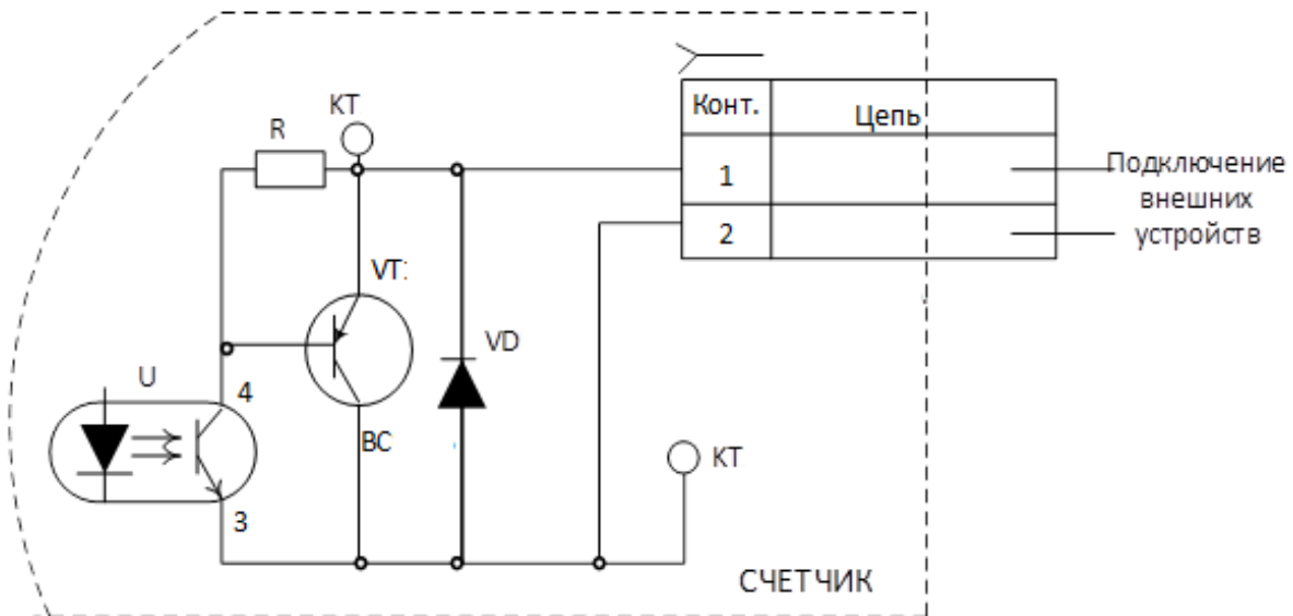
Рисунок 4 - Тип электрических импульсных выходов счетчика
